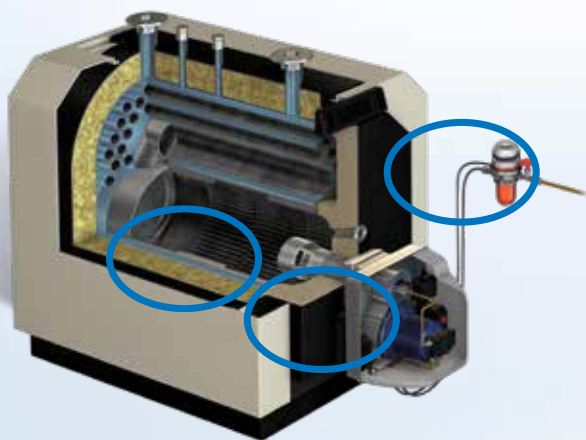
Heizölkessel
